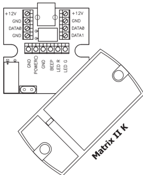
6. Подключение контроллера Matrix II K к адаптеру Z-2 Base
