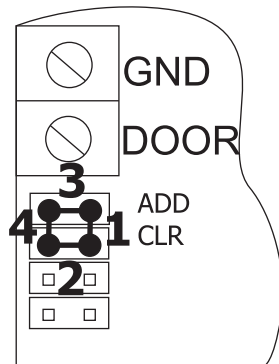
Рис.6 Положения переключки
