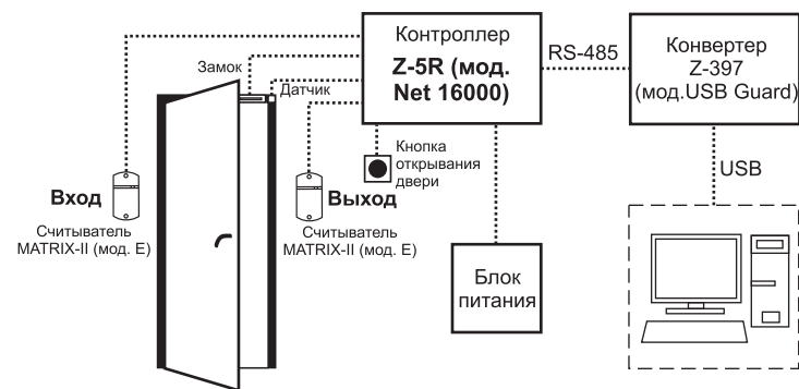
Рис.1 Схема СКУД с контроллером Z-5R (mod. Net 16000)
