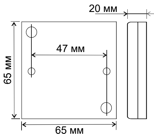
Рис.7 Внешний вид корпуса и габаритные размеры
